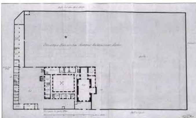
4. kép A hatvani kapucinus kolostor és templom földszinti alaprajza Joseph Thalherr kamarai mérnök rajza (1796) MNL OL T 62 1195/2
