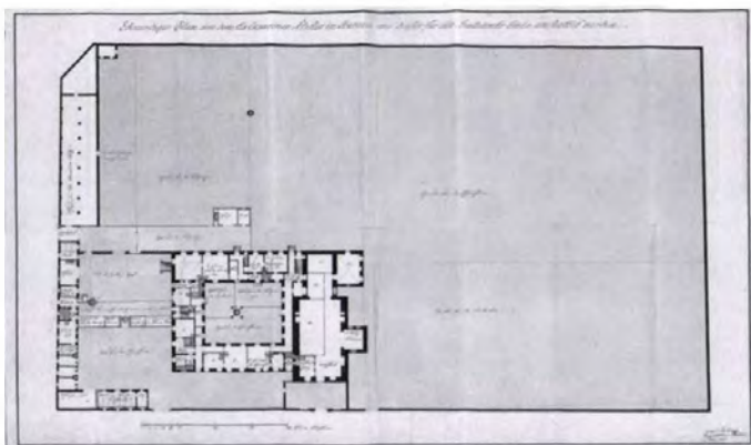
5. kép A hatvani kapucinus kolostor és templom földszinti helyiségeinek tervezett átalakítása sóhivatallá Joseph Thalherr kamarai mérnök rajza (1796) MNL OL T 62 1195/3
